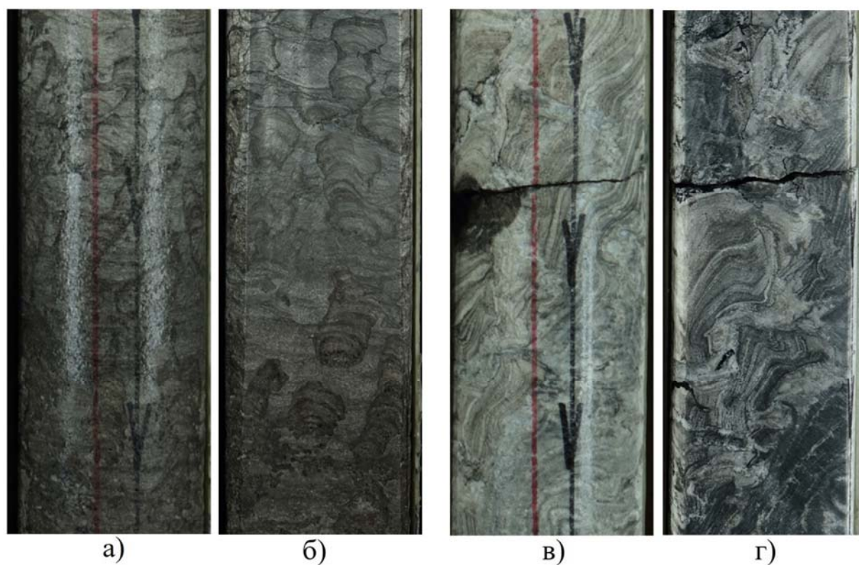
Рис. 2. Фотографии кернового материала: а) строматолитовый доломит (нераспиленный керн); б) столбчатые строматолиты в прижизненном положении (продольный спил керна); в) карбонатная брекчия (нераспиленный керн); г) карбонатная брекчия с обломками строматолитов (продольный спил керна)
