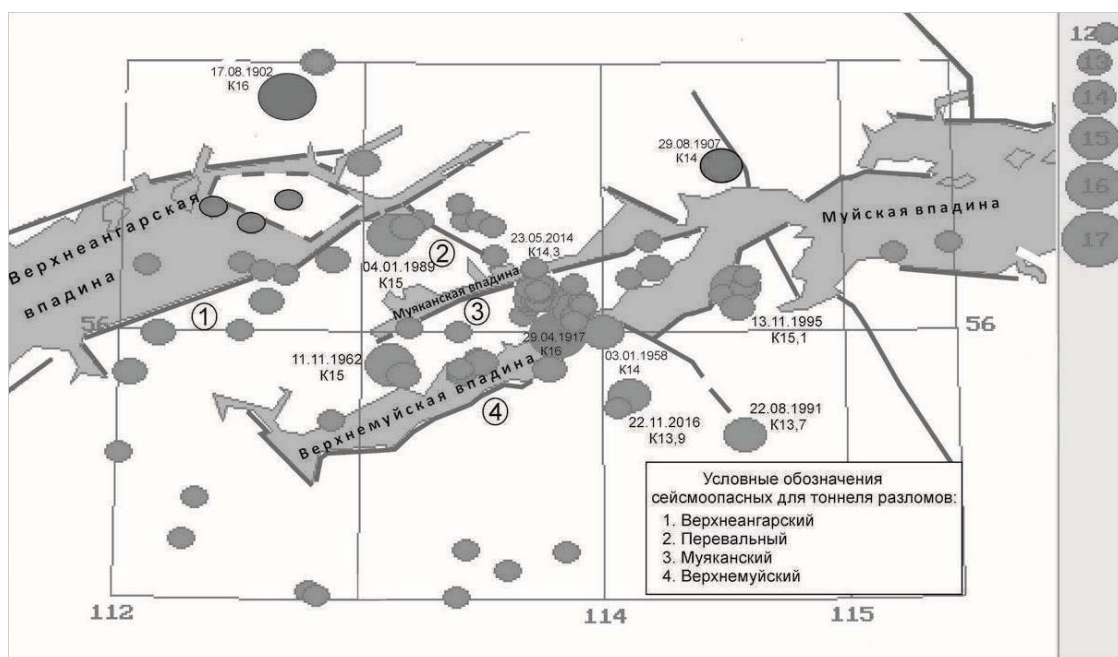
Рис. 1. Сейсмотектоническая схема строения межвпадинной перемычки между Верхнеангарской и Муйской рифтовыми впадинами и расположение эпицентров сильных землетрясений с K_p = 12-17 ( M \geq 4,5 )
