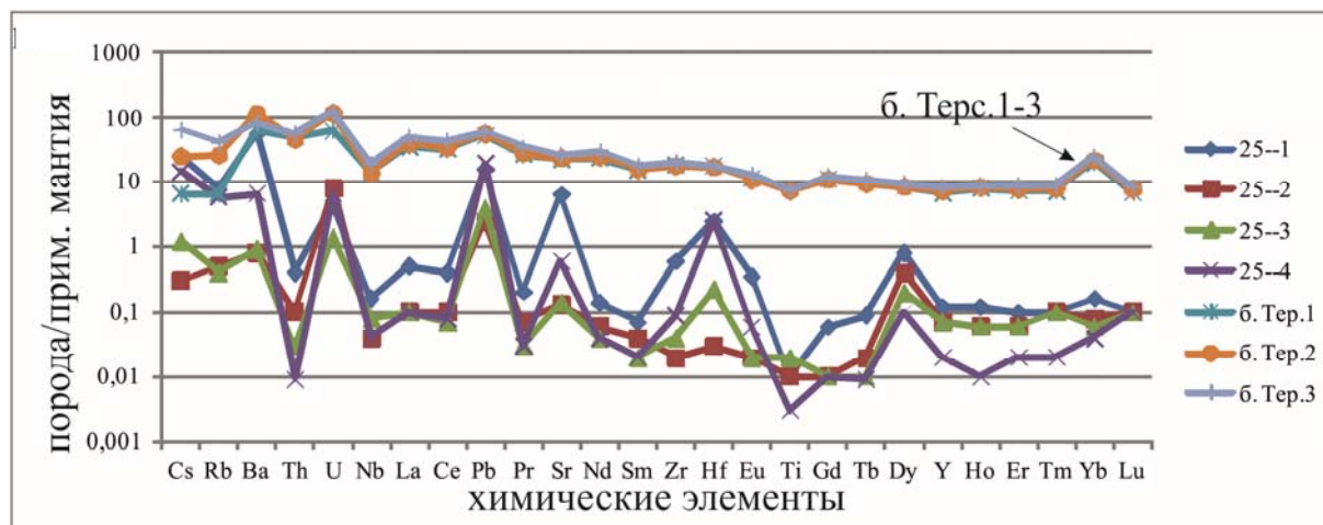
Рис. 4. Нормированные на примитивную мантию графики распределения редкоземельных элементов в образце 25 и базальта (б. Терс.1-3) [Sun, McDonough, 1989]
