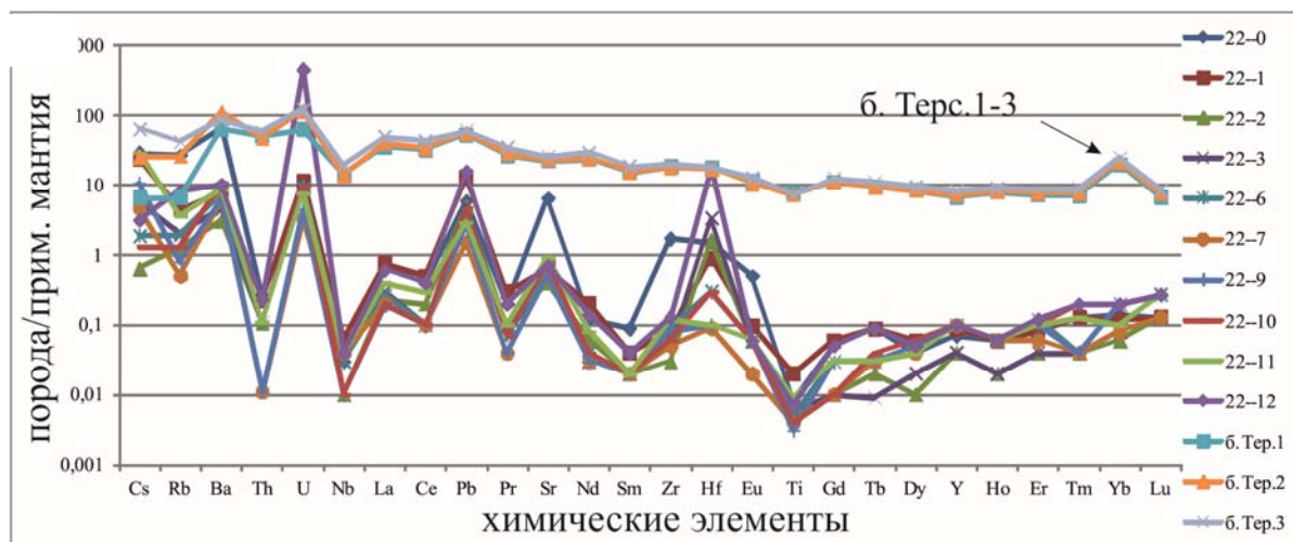
Рис. 3 Нормированные на примитивную мантию графики распределения редкоземельных элементов в образце 22 и базальта (б. Терс.1-3) [Sun, McDonough, 1989]
