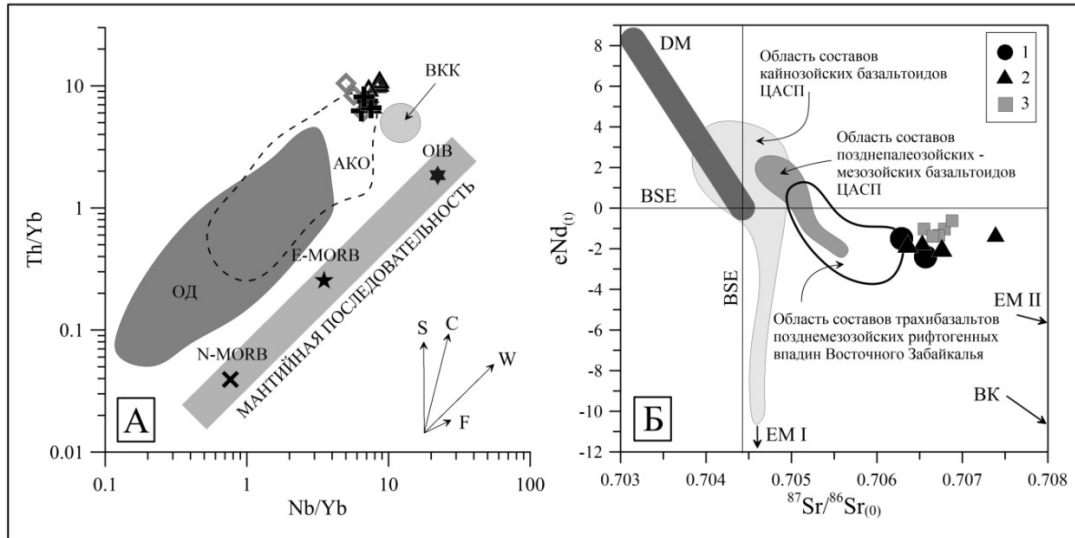
Рис. 2. Диаграммы \text{Th/Yb} - \text{Nb/Yb} и \epsilon\text{Nd}(t) - {}^{87}\text{Sr}/{}^{86}\text{Sr} для позднемезозойских вулканитов Нерчинской впадины
