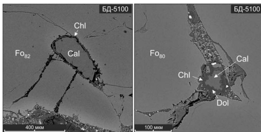
Рис. 3. Включения карбонатных фаз в оливинах из базанитов вулкана Бодь-уул
